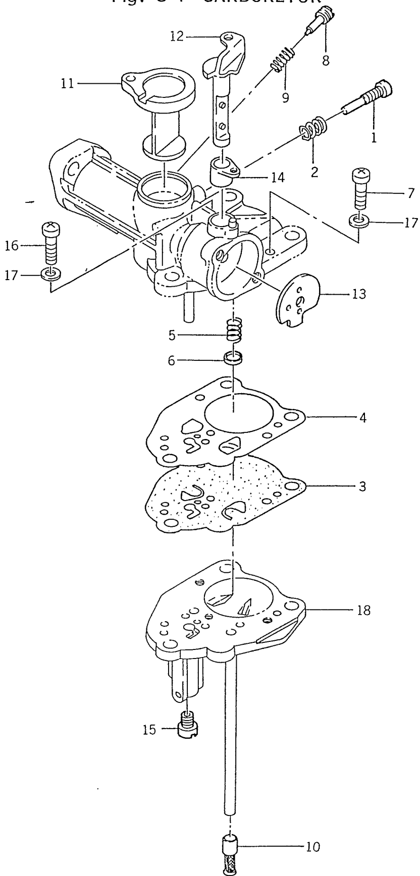
Fig. C-1 CARBURETOR
